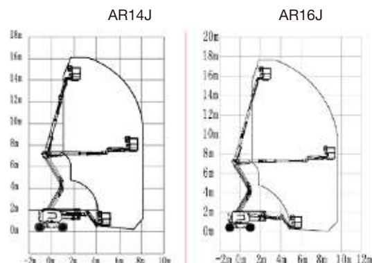
Pracovní rozsahy
